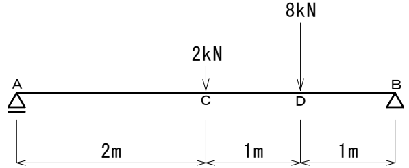
図2 単純梁
