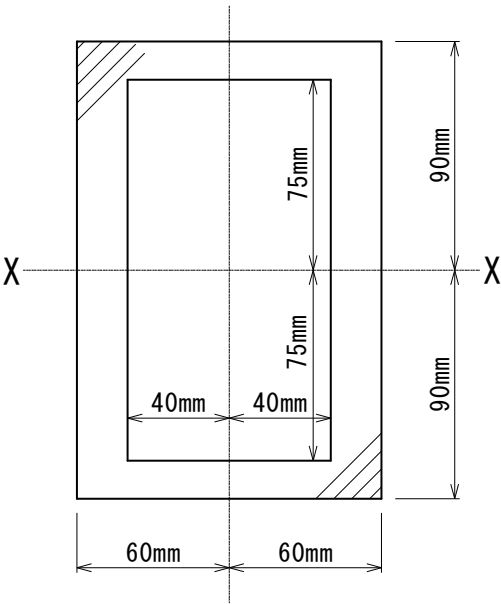
図1 断面
