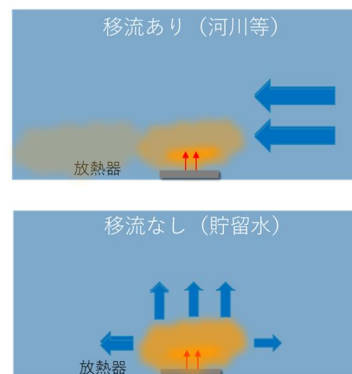
図2 河川等(上図)と貯留水(下図)の熱拡散の違い
