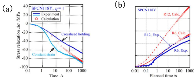
応力緩和試験
