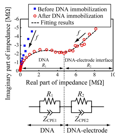
図 3. DNA の電気的な特性
