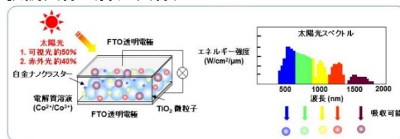
図3 金属ナノクラスター型太陽電池の構成図
