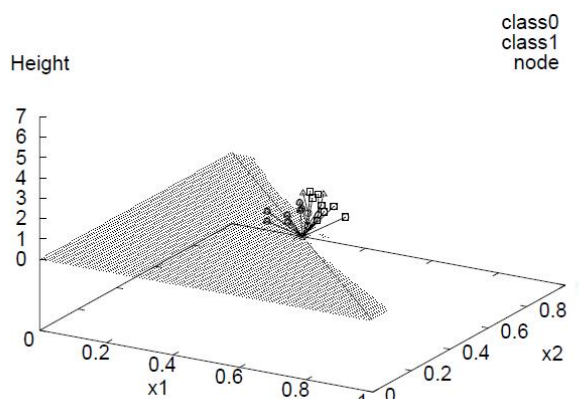
枝刈り後の自己組織化ニューラル木
