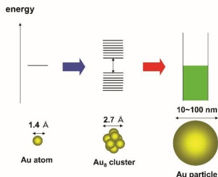
図1 Jellium の理論モデルより求められた金ナノクラスターの分子軌道モデル
