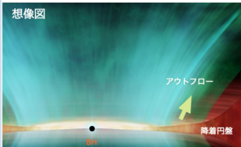
図 1 アウトフローの想像図。中心にある BH へプラズマ回転円盤状（降着円盤と呼ばれる）になりながら落ち込む。その一部がアウトフロー（図の緑）として外部へ噴出される。
